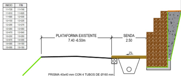
S-7 (SECCIÓN SENDA CON MURO DE PERPIAÑO)
