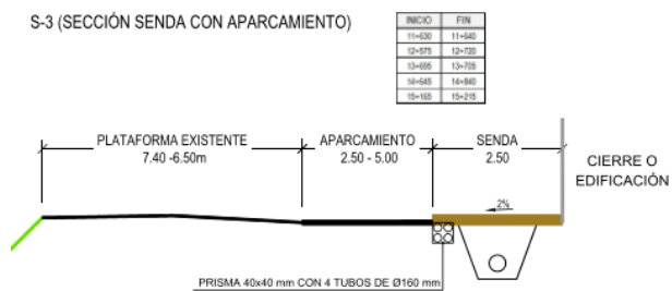
S-3 (SECCIÓN SENDA CON APARCAMIENTO)
