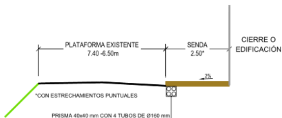
S-1 (SECCIÓN REPOSICIÓN DE ACERA EXISTENTE P.K. 14+195-14+645)
