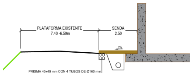
S-8 (SECCIÓN SENDA CON MURO DE HORMIGÓN P.K. 13+875-13+895)
